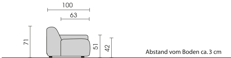
Seitenansicht Elemente
